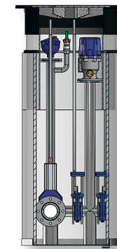
ARMARE-TEC Entleerungshydrant
