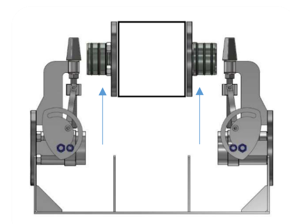
FLEXClean System Armatur – Messeinrichtung mit Buchsen ausheben
