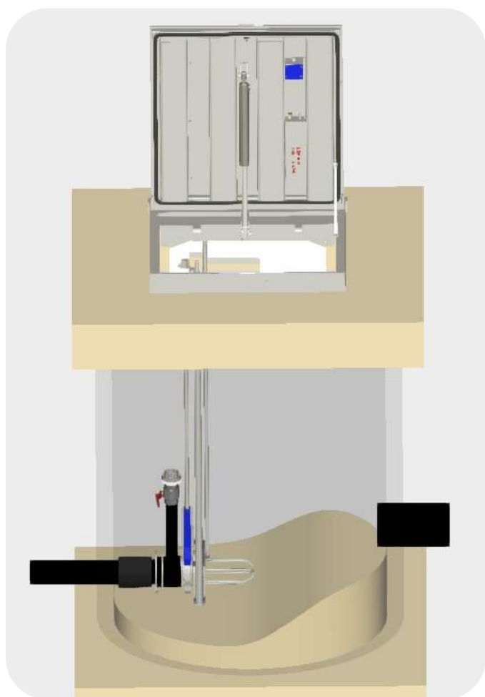
KOMPACT Schacht Druckenschacht FLEXClean 3D Darstellung mit Schachtboden-Etagierung
