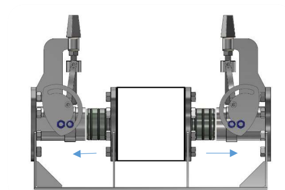
FLEXClean System wird betätigt - Hülsen zurückgeschoben
