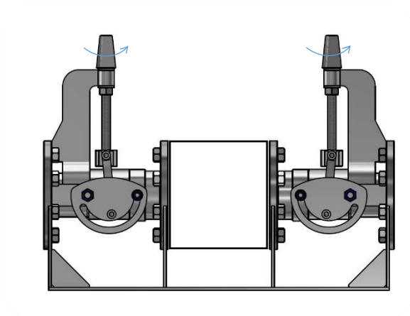
FLEXClean System in Betrieb
