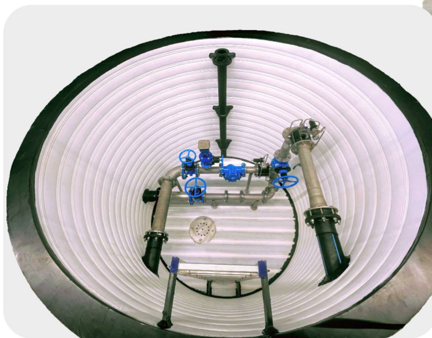
KOMPACT SCHACHT, WZ-BEV-DMS Druckminderer-Schacht inkl. Sicherheits-/Druckhalteventil – Ausstattung nach Kundenwunsch
