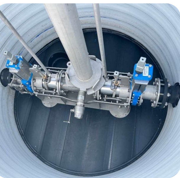
FLEXClean System - Spül- und Molchsäule mit FLEX-DREH-Flansch entnehmen
