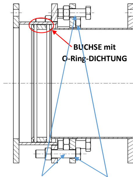
Feststell-Schrauben Distanzschrauben
