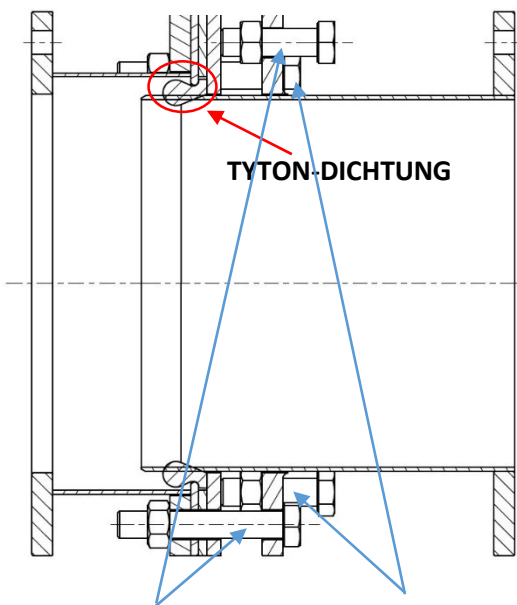
Feststell-Schrauben Distanzschrauben
